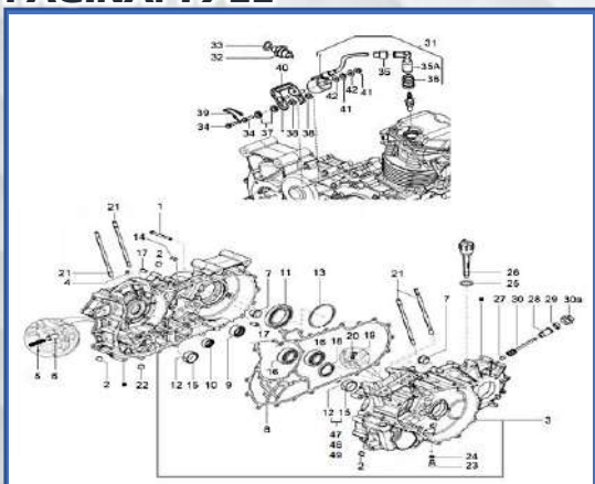
LAMINA-9 CAJA DE CIGÜEÑAL PAGINA: 19-22
