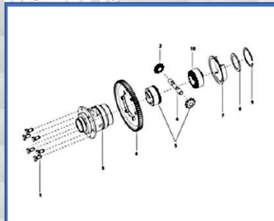
LAMINA-5 ENGRANES DE DIFERENCIAL PAGINA: 9-10
