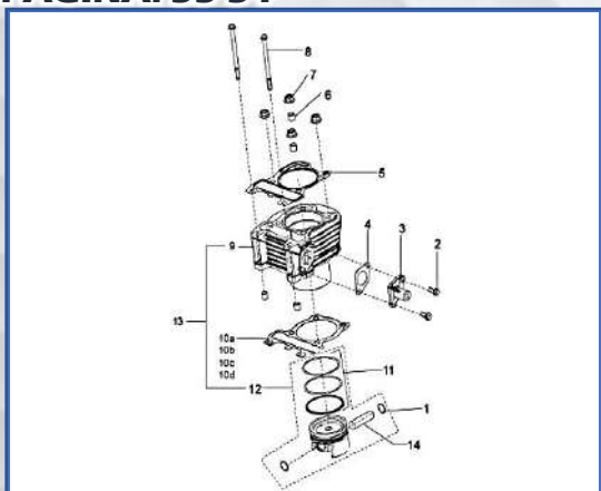
LAMINA-15 CILINDRO, PISTÓN Y ANILLOS PAGINA: 33-34
