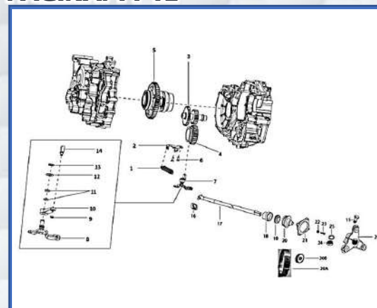
LAMINA-6 CONJUNTO DE DIFERENCIAL PAGINA: 11-12
