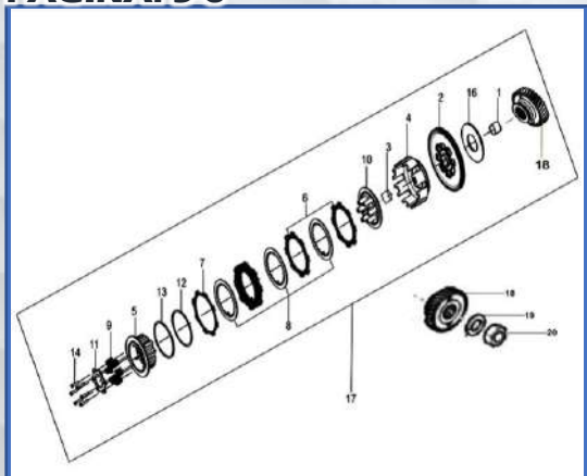
LAMINA-3 CONJUNTO DE CLUTCH PAGINA: 5-6
