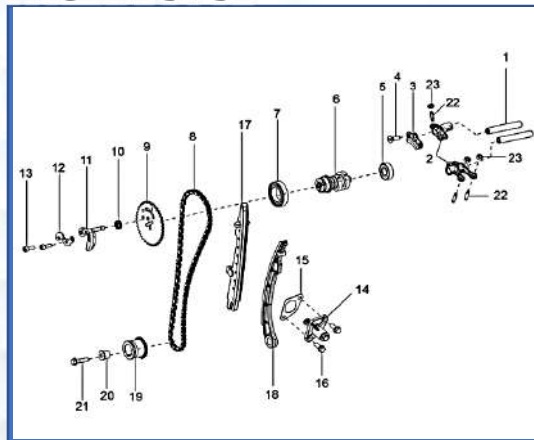
LAMINA-14 COMPONENTES DE PUESTA A TIEMPO PAGINA: 31-32
