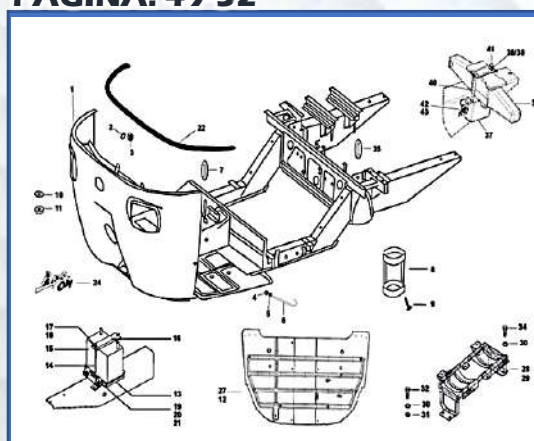
LAMINA-22 CARROCERIA/SOPORTE DE BATERIA/SUJETADOR DE BATERIA PAGINA: 49-52
