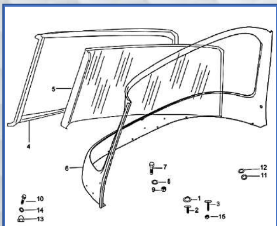
LAMINA-21 PARABRISAS/ MARCO Y GOMA PAGINA: 47-48
