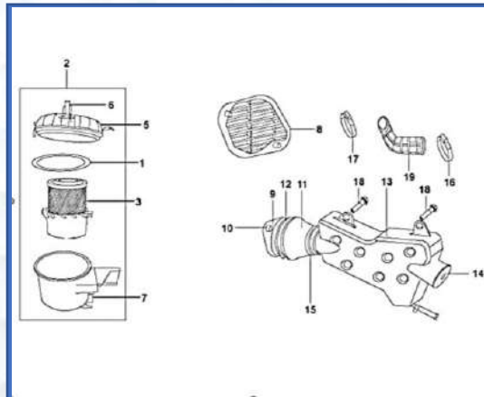
LAMINA-8 CONJUNTO DE FILTRO DE AIRE PAGINA: 17-18
