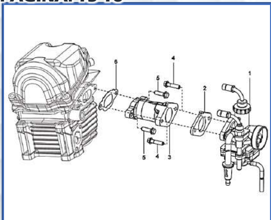
LAMINA-7 COPLE DE ADMISION Y CARBURADOR PAGINA: 13-16
