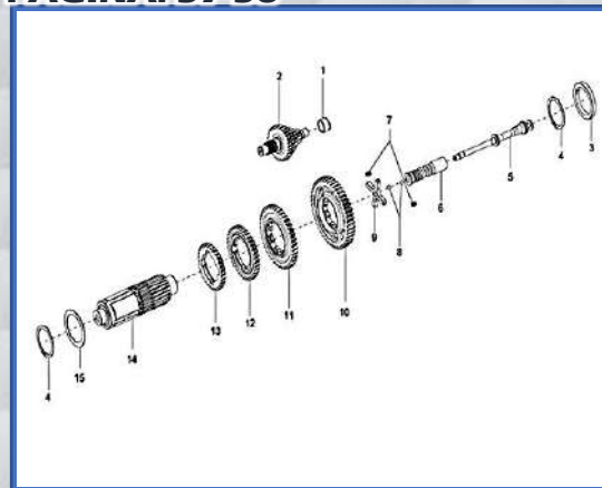
LAMINA-17 GRUPO DE ENGRANAJES CAJA VELOCIDADES PAGINA: 37-38
