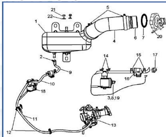
LAMINA-20 TANQUE , FILTRO, MANGUERAS DE COMBUSTIBLE – CITY GLP PAGINA: 45-46
