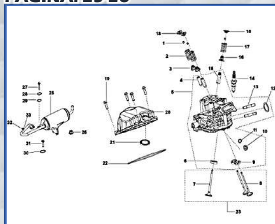
LAMINA-11 CABEZA DE CILINDRO PAGINA: 25-26
