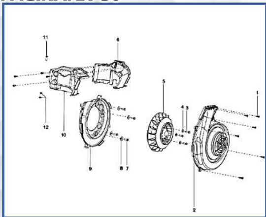
LAMINA-13 COMPONENTES DE CIRCUITO DE ENFRIAMIENTO PAGINA: 29-30
