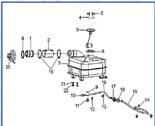
LAMINA-19 TANQUE , FILTRO, MANGUERAS DE COMBUSTIBLE PAGINA: 43-44
