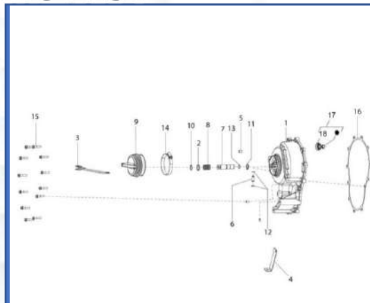
LAMINA-2 TAPA DE CLUTCH PAGINA: 3-4
