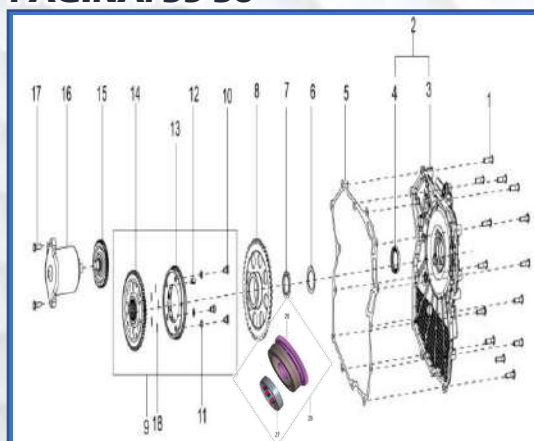
LAMINA-16 COMPONENTES DE ENCENDIDO PAGINA: 35-36
