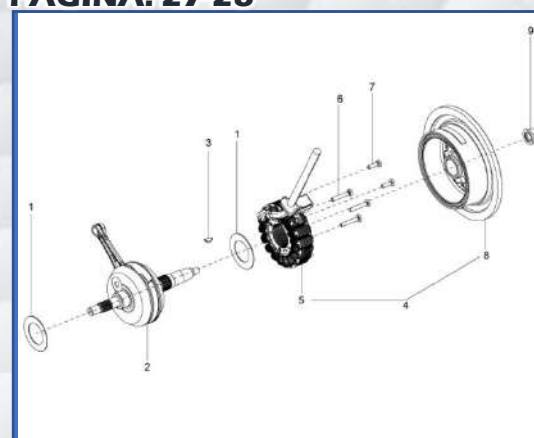
LAMINA-12 CONJUNTO DE CIGÜEÑAL PAGINA: 27-28
