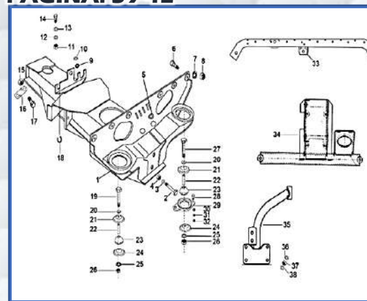
LAMINA-18 GRUPO DE SOPORTES DE MOTOR PAGINA: 39-42
