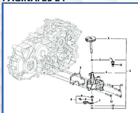
LAMINA-10 CAJA DE SELECTOR PAGINA: 23-24
